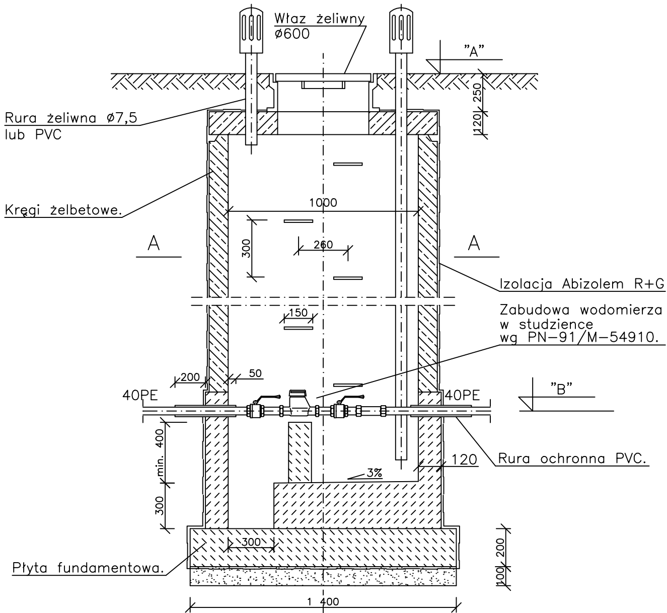
Przekrój A-A
